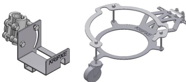
SOPORTE MANGUERA AIRLESS COD.009150-3700
